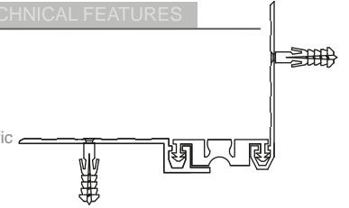
AR151-051 KÖŞE DETAYI AR151-051 CORNER DETAIL
