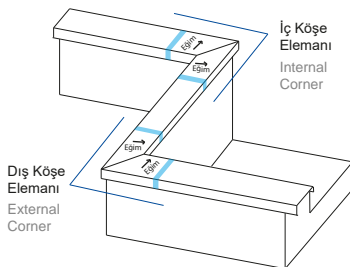
Dış Köşe ve İç Köşe Elemanı (External and Internal Corner Parts)
