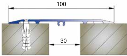
AR100 ZD (Zemin) AR100 ZD (Floor)
