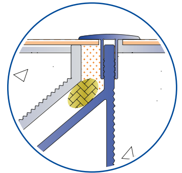
Zemin geçiş profili Floor trim profile
