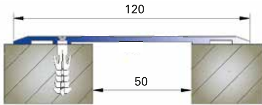
AR120 ZD (Zemin) AR120 ZD (Floor)
