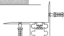
AR171-035 KÖŞE DETAYI AR171-035 CORNER DETAIL
