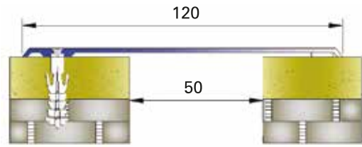
AR120 DT (Duvar Tavan) AR120 DT (Wall / Ceiling)
