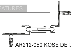
AR212-050 KÖŞE DETAYI AR212-050 CORNER DETAIL
