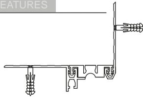
AR151-050 KÖŞE DETAYI AR151-050 CORNER DETAIL
