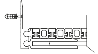
AR303-150 KÖŞE DETAYI AR303-150 CORNER DETAIL
