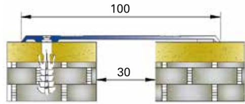
AR100 DT (Duvar Tavan) AR100 DT (Wall / Ceiling)
