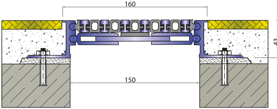
AR303-150 KÖŞE DETAYI AR303-150 CORNER DETAIL
